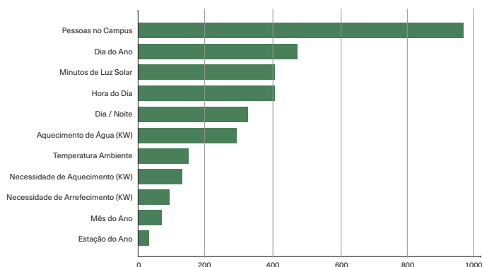
Valor Shapley Absoluto Médio (Impacto Médio na Magnitude do Valor de Saída do Modelo)
